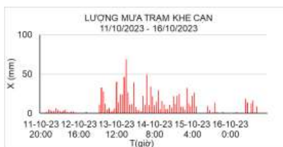
Hình 5: Lượng mưa trạm Khe Cạn 2023
