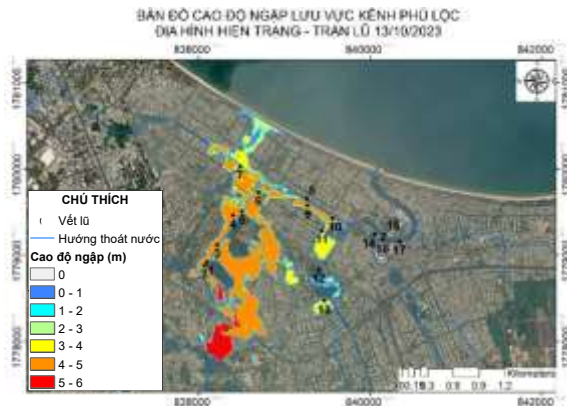
Hình 11: Cao độ ngập hiện trạng - 13/10/2023
