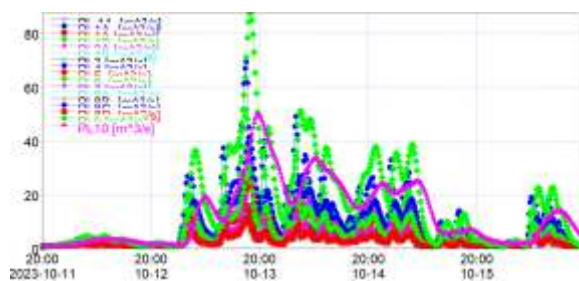
Hình 17: Biên Q_{P=10\%} các tiểu lưu vực
