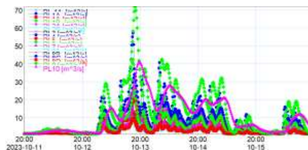
Hình 18: Biên Q_{P=20\%} các tiểu lưu vực
