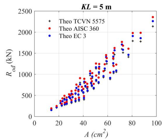
Hình 6. Sức kháng nén xét theo điều kiện ổn định
