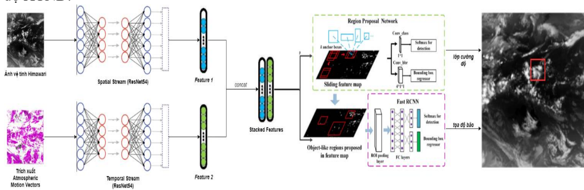
Hình 7. Cấu trúc mạng không - thời gian để nhận dạng XTNĐ.
