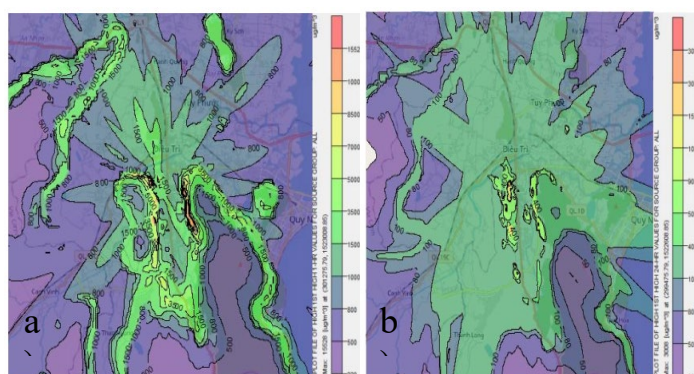
Hình 20. Bản đồ lan truyền CO trong a) 1 giờ b) 8 giờ cho nhà máy theo KB3.
