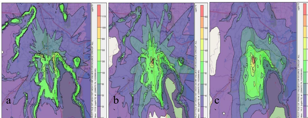
Hình 11. Bản đồ lan truyền \text{NO}_2 trong a) 1 giờ b) 24 giờ c) trung bình năm cho nhà máy theo KB1.
