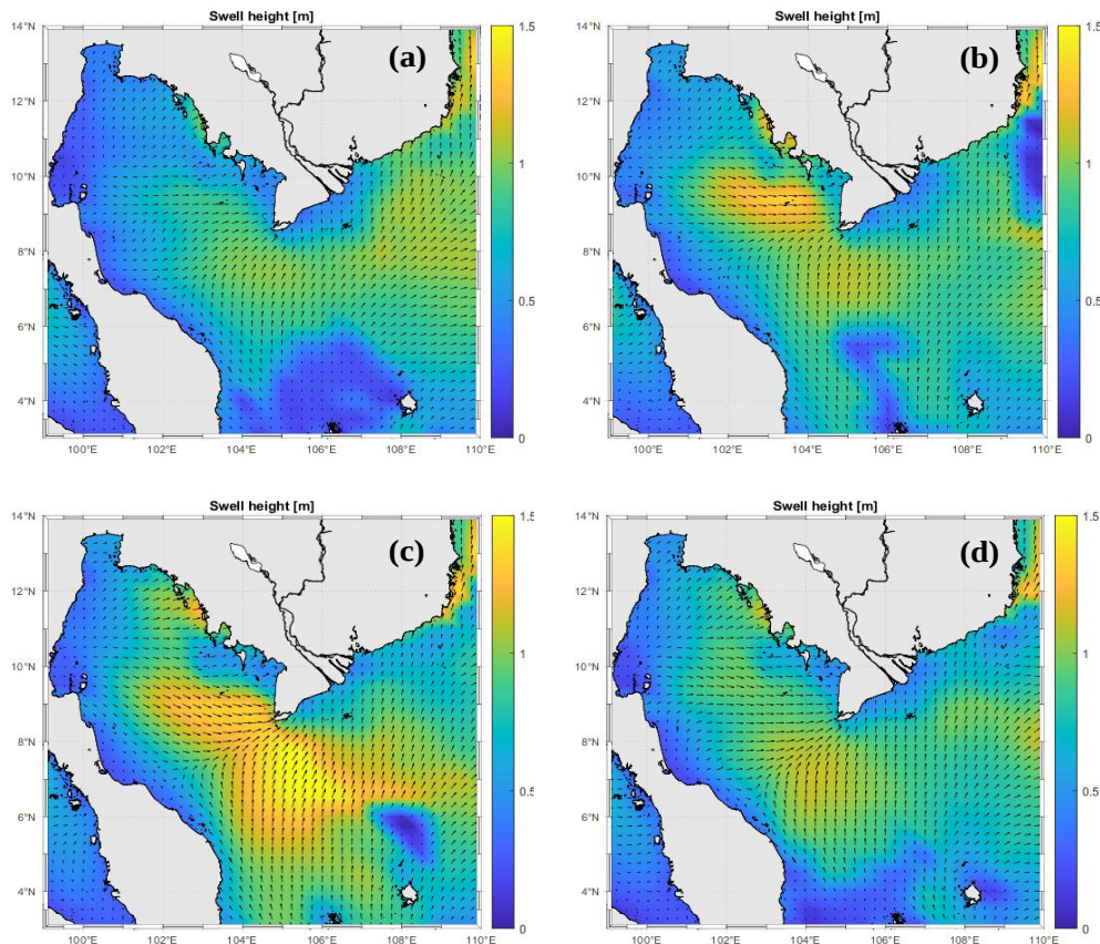
Hình 12. Phân bố trường sóng lừng tại các thời điểm trước, trong và sau thời gian xuất hiện đợt triều cường kèm theo sóng lớn tại ven biển Tây Cà Mau: (a) 13 ngày 31/7/2019; (b) 13 giờ ngày 02/8/2019; (c) 13 giờ ngày 03/8/2019; (d) 13 giờ ngày 04/8/2019.
