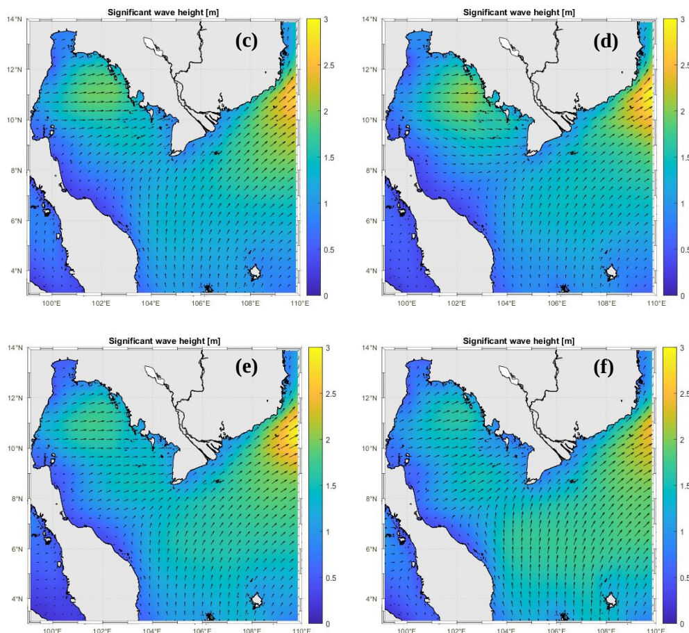
Hình 9. Phân bố trường sóng có nghĩa ( H_{Sig.} ) tại các thời điểm trước, trong và sau ngày xuất hiện triều cường cao kèm theo sóng lớn tại ven biển Tây Cà Mau: (a) 13h ngày 29/7/2019; (b) 13 giờ ngày 31/7/2019; (c) 13h ngày 02/8/2019; (d) 13h ngày 03/8/2019; (e) 13h ngày 04/8/2019; (f) 13h ngày 04/8/2019.
