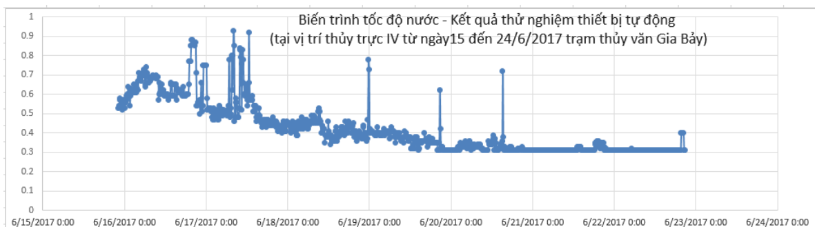
Hình 5. Biến trình tốc độ nước tại thủy trực đại biểu – đo thử nghiệm tại trạm thủy văn Gia Bảy.
