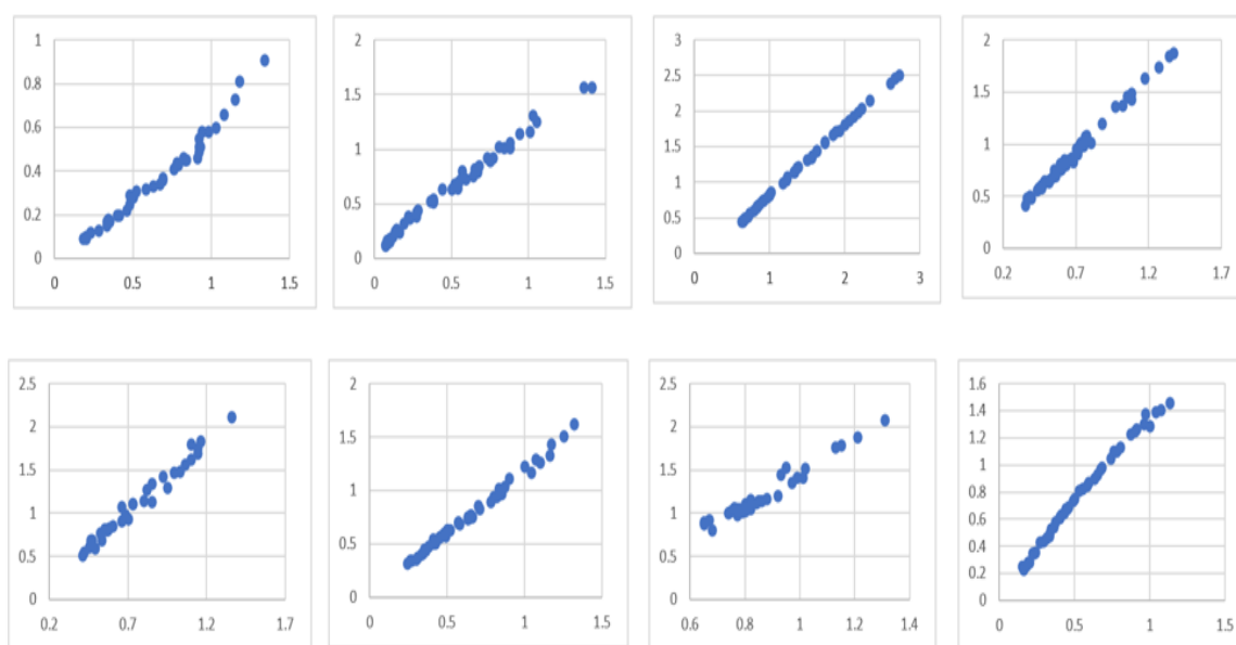
Hình 6. Biểu đồ tương quan V_{tb} = f(V_m) tại thủy trực đại biểu của các trạm thủy văn – lần lượt từ trái sang phải, từ trên xuống dưới là trạm Bảo Yên, Gia Bảy, Lào Cai, Hòa Duyệt, Sơn Diệm, Yên Thượng, Giang Sơn, Phước Hòa.
