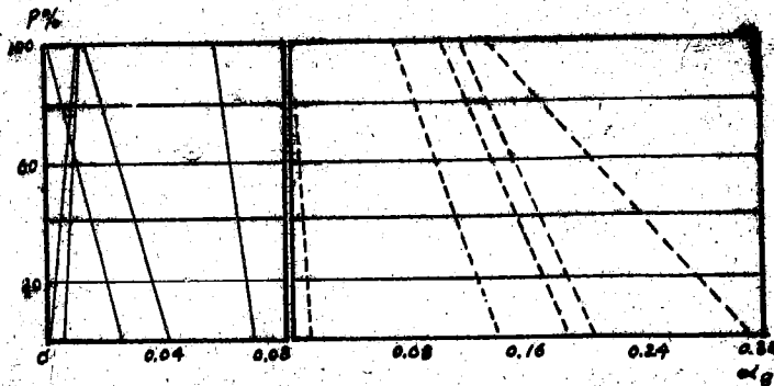
Hình 3 - So sánh hệ số dòng chảy sườn dốc \alpha_p với mức độ khai hoang (Bãi hoang : p = 0\% ; đã khai hoang : p = 100\% ).
