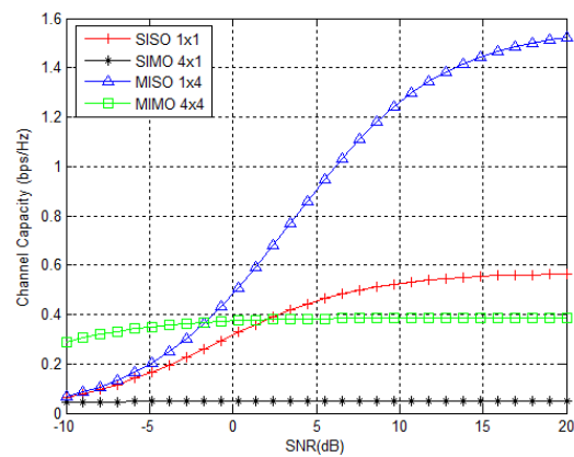
Hình 8. Dung lượng hệ thống với tương quan thu lớn nhất
