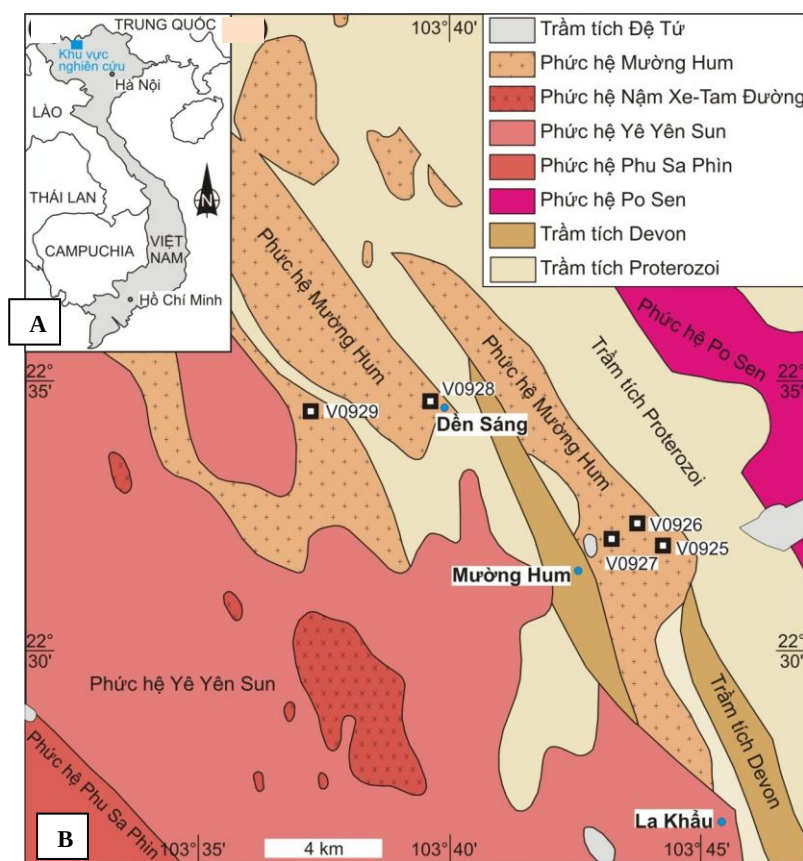
Hình 1. Sơ đồ các thành tạo magma xâm nhập khu vực Phan Si Pan, Tây Bắc Việt Nam và vị trí lấy mẫu (theo tài liệu bản đồ tỷ lệ 1:200.000 tờ Kim Bình-Lào Cai [4])
