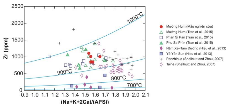
Hình 7. Nhiệt độ bão hòa zircon của granite kiềm khối Mương Hum [8]
