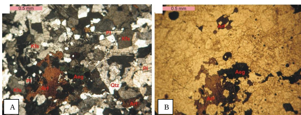
Hình 3. Mẫu lát mỏng V0927 của granite kiềm khối Mùòng Hum: (A) ảnh lát mỏng dưới 2 nicol, (B) ảnh lát mỏng dưới 1 nicol. Aeg=Aegirine, Arf= Arfvedsonite, Kfs= Alkaline feldspar, Pl= Plagioclase, Qtz= Thạch anh
