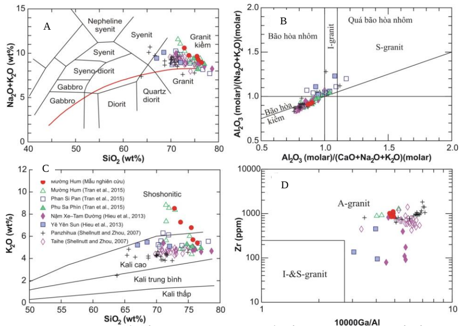
Hình 4. (A) SiO_2 -( Na_2O+K_2O ): biểu đồ phân loại đá [14]; (B) Biểu đồ tương quan giữa chỉ số kiềm và chỉ số bão hòa nhôm phân chia các loại magma [5]; (C) K_2O - SiO_2 : biểu đồ tương quan hàm lượng potassium [1]; và (D) Zr - 10,000 \times Ga/Al : biểu đồ phân loại granite [12]
