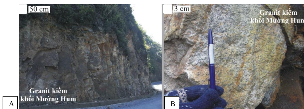
Hình 2. Đặc điểm địa chất các thành tạo granite kiềm khối Mùòng Hum: (A) Granite kiềm khối Mùòng Hum bị nén ép dập vỡ; (B) Granite kiềm khối Mùòng Hum màu xám trắng, hạt thô, dạng dải định hướng
