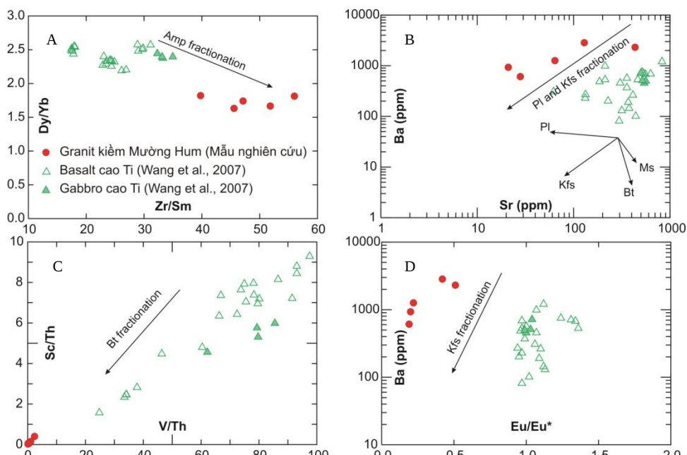
Hình 8. (A) Zr/Sm-Dy/Yb, (B) Sr-Ba, (C) V/Th-Sc/Th, và (D) Eu/Eu*-Ba: biểu đồ so sánh sự phân dị kết tinh của granite kiềm khối Mương Hum với các đá mafic cao Ti Sông Đà. Amp = amphibole, Pl = plagioclase, Kfs = alkaline feldspar, Bt = biotite, Ms = Muscovite
