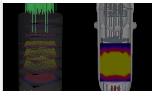
Hình 4. Giao diện hệ mô phỏng lõi lò OPR1000 hiển thị 3D
