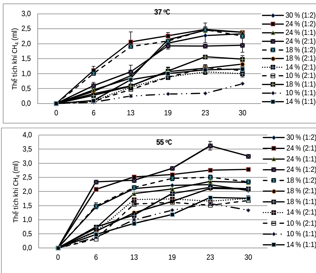
Hình 1. Ảnh hưởng của nhiệt độ đến thể tích khí methane tạo thành theo thời gian phản ứng ở nhiệt độ 37 °C (Hình A) và 55 °C (Hình B), với các nồng độ rắn và các tỷ lệ phối trộn khác nhau. Sai số thể hiện trên hình là \pm SD
