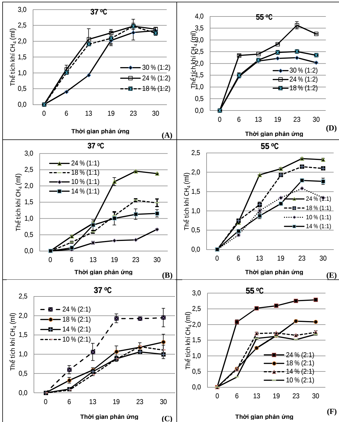
Hình 2. Ảnh hưởng của % khối lượng rắn đến thể tích khí methane tạo thành theo thời gian ở nhiệt độ 37 °C [tỷ lệ phối trộn 1:2 (Hình A), 1:1 (Hình B), 2:1 (Hình C)] và ở nhiệt độ 55 °C [tỷ lệ phối trộn 1:2 (Hình D), 1:1 (Hình E), 2:1 (Hình F)]. Sai số thể hiện trên hình là \pm SD
