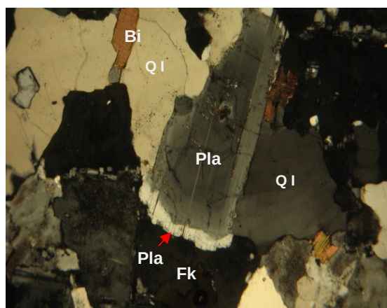
Hình 22. Granite biotite pha 2. Orthite cấu tạo đôi trắng. Lát mỏng XY06/2; 1Ni + ; 3.3x10 x .
