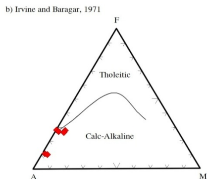
Hình 2. Biểu đồ phân loại granitoid khối Xá Yù theo Lemaître 1989; Irvine & Baragar, 1971
