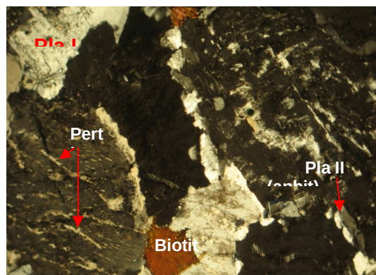
Hình 13. Granite biotite pha 1 plagiocla II. Lát mỏng XY010; 2Ni + ; 3.3x5 x .
