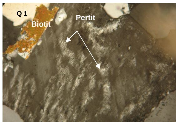
Hình 15. Granite biotite pha 1. Potassium feldspar cấu tạo pertite. Lát mỏng XY05; 2Ni + ; 3.3x5X
