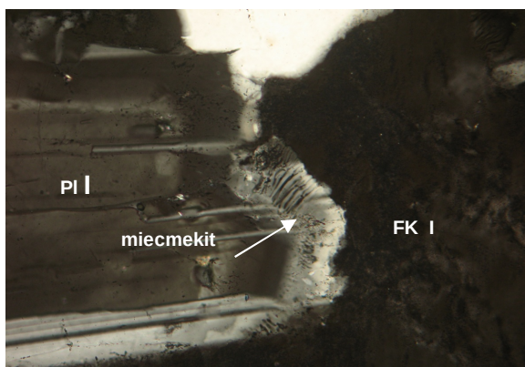
Hình 12. Granite biotite pha 1. Kiến trúc micmekite. Lát mỏng XY11/1; 2Ni + ; 3.3x10X.
