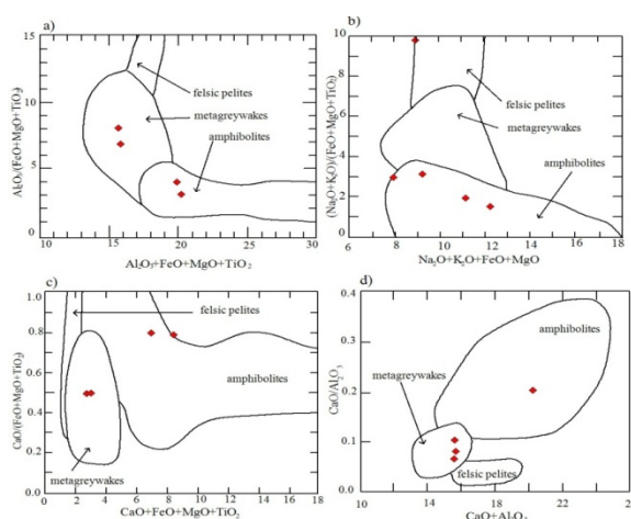
Hình 11. Nguồn gốc thành tạo granitoid khối Xả Yủ theo Patino Douce 1999
