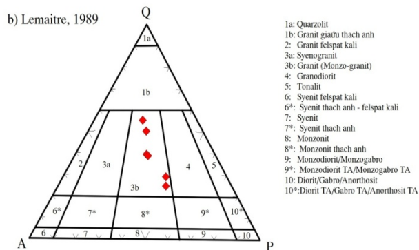
Hình 1. Biểu đồ phân loại granitoid khối Xá Yù Lemaître 1989; Irvine & Baragar, 1971
