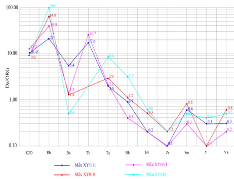
Hình 7. Biểu đồ các nguyên tố vi lượng của granitoid khối Xả Yủ granitoid được chuẩn hóa theo granite sông núi giữa đại dương với Chondrite theo (ORG) theo Pearce J.A.et al., 1984
