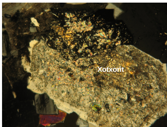
Hình 21. Granite biotite pha 2. Plagioclas bị xotxorit hóa hoàn toàn. Lát mỏng XY016/1; 2Ni + ; 3.3x10 x .
