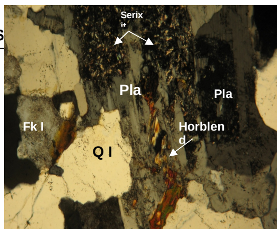
Hình 18. Granite biotite pha 2. Plagioclas cấu tạo đôi, L m XY06/1; 2Ni + ; 3.3x10 x .318.
