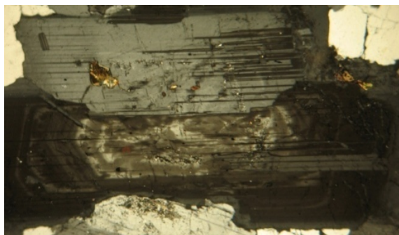
Hình 16. Granite biotite pha 1. Plagiocla cấu tạo đối. Lát mỏng XY07; 2Ni + ; 3.3x5 x
