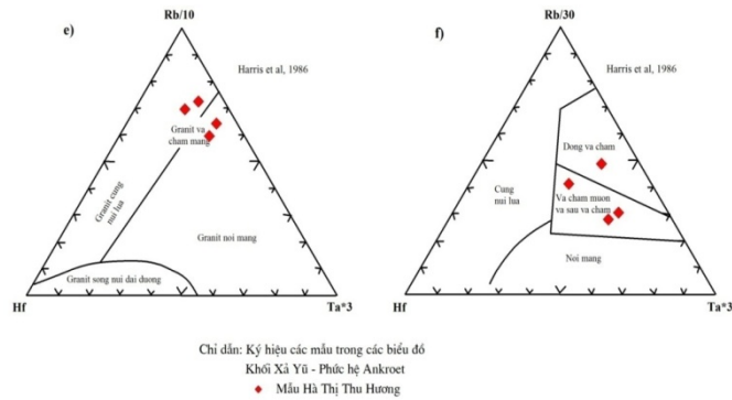
Hình 10. Biểu đồ phân chia bối cảnh kiến tạo granitoid khối Xả Yù Harris et al, 1986
