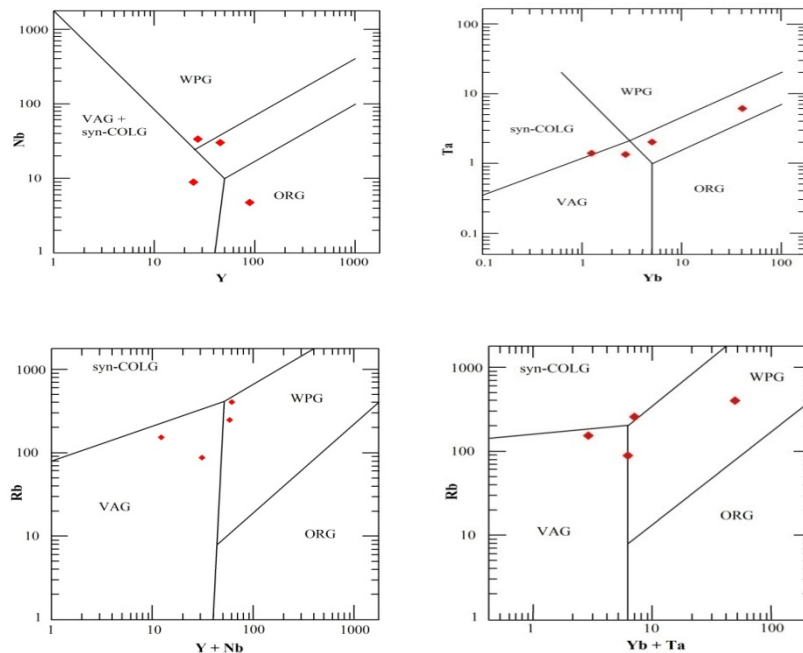
Hình 9. Biểu đồ phân chia bối cảnh kiến tạo granitoid khối Xả Yũ theo Pearce 1984 (a,b,c,d);
