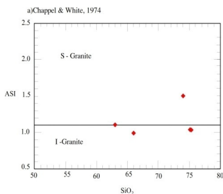
Hình 5. Chappel và White 1974
