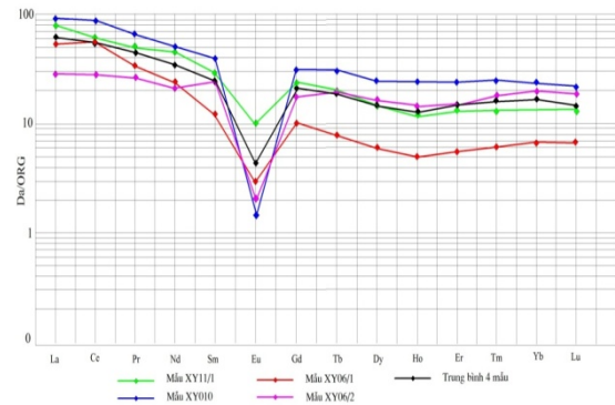
Hình 8. Biểu đồ các nguyên tố REE của khối Xả Yủ được chuẩn hóa Boynton, 1984
