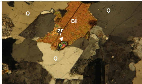
Hình 17. Granite biotite pha 1. zircon (Zr) trong biotite (Bi) ; Lát mỏng XY05/1; 2Ni + ; 3.3x10X.
