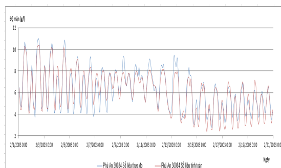
Hình 11. Kết quả hiệu chỉnh độ mặn tại trạm Phú An
