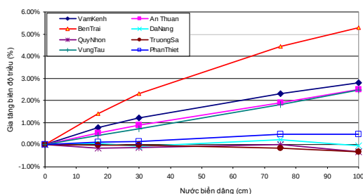
Hình 2. Ảnh hưởng nước biển dâng tới biên độ triều
