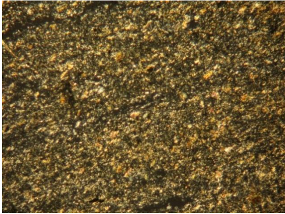
Hình 4. Sét bột kết, XT04, 2N+ 40X. Vẩy serixit có màu vàng nhạt
