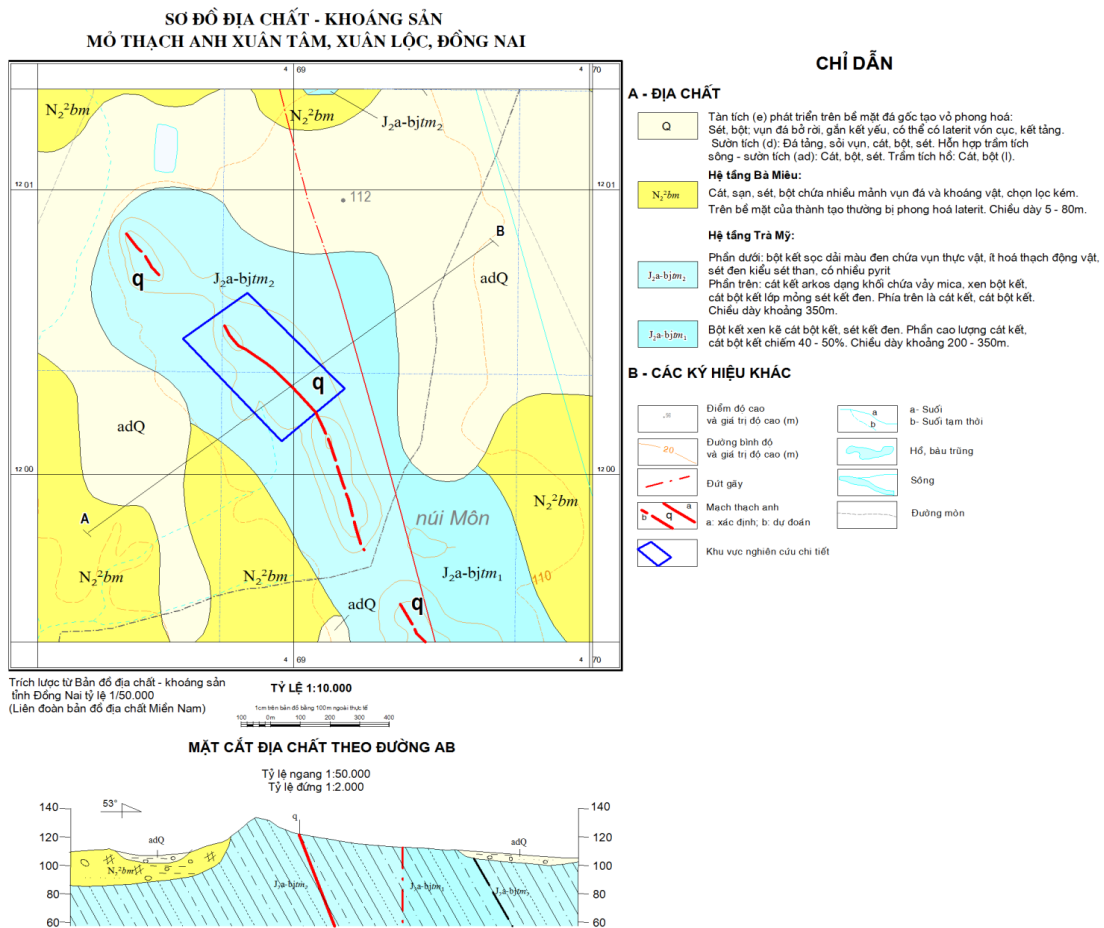
Hình 1. Sơ đồ địa chất – khoáng sản mỏ thạch anh Xuân Tâm, Xuân Lộc, Đồng Nai
