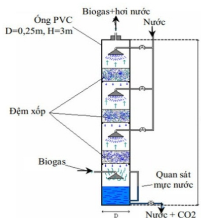
Hình 2. Lọc \text{CO}_2 bằng nước [8]
